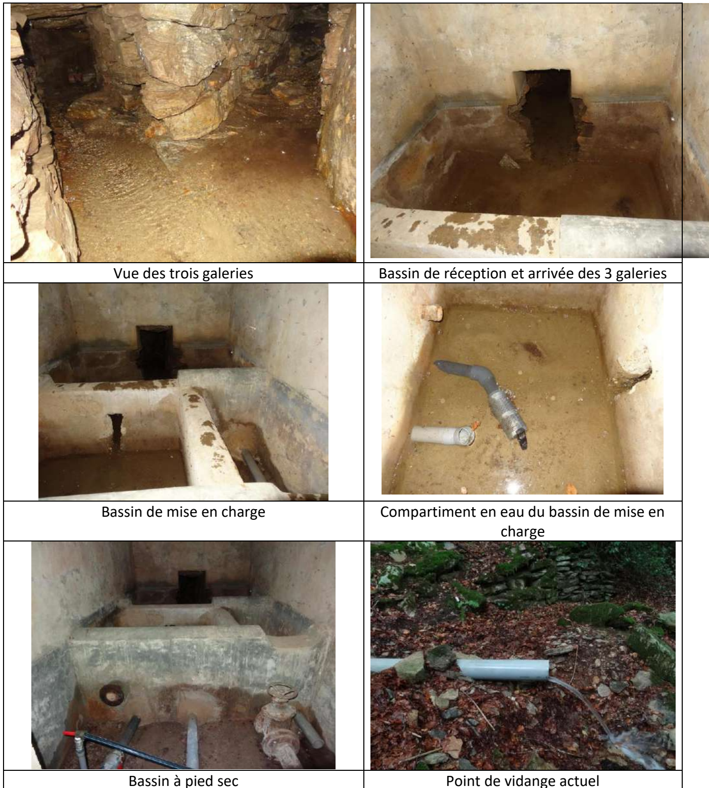
Figure 8 : planches photographiques du captage Peyris – vue intérieure
