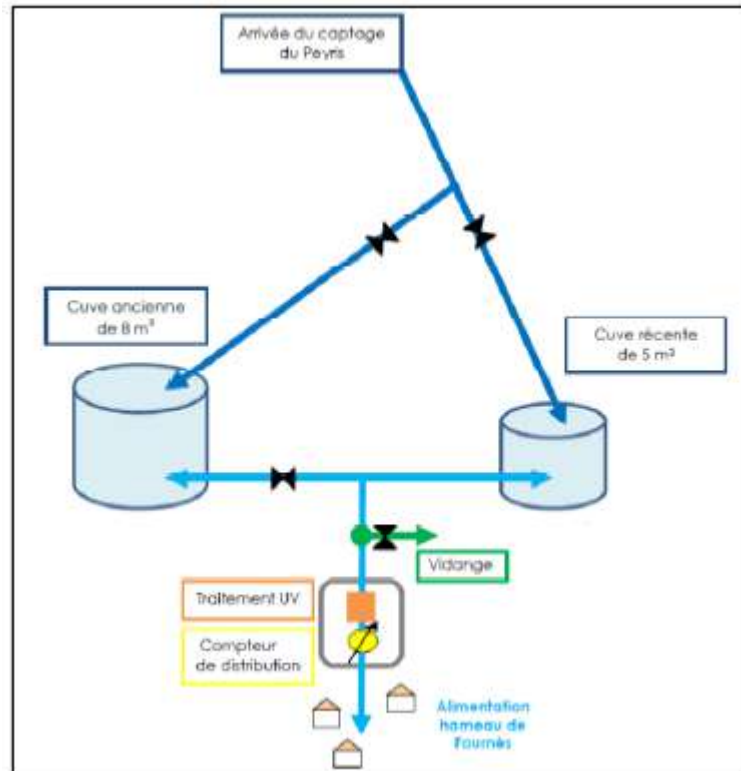
Figure 9 : Schéma du réseau de distribution (source Conseil Général 11)
