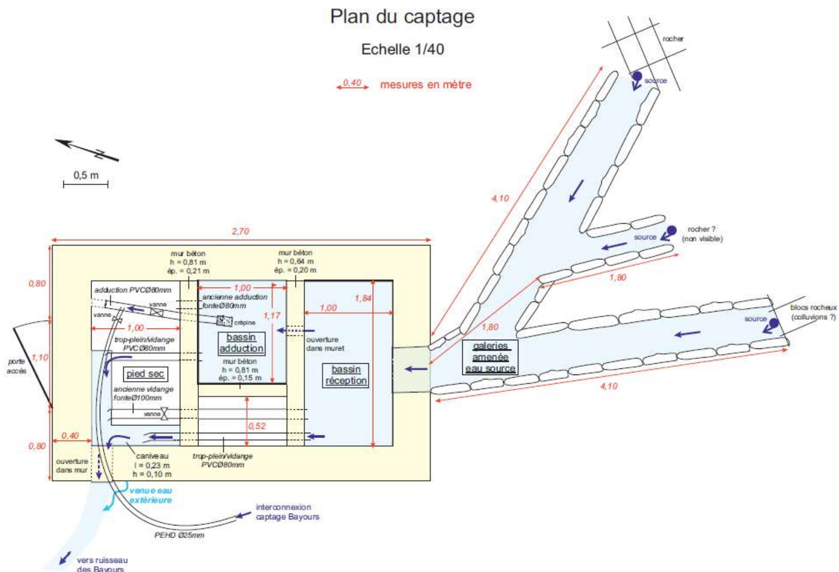
Figure 7 : Plan schématique du captage de la source Peyris (source hydrogéconsult)
