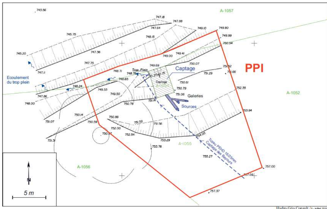
Figure 14 : Proposition de tracé du bureau d'étude – sur plan géomètre
