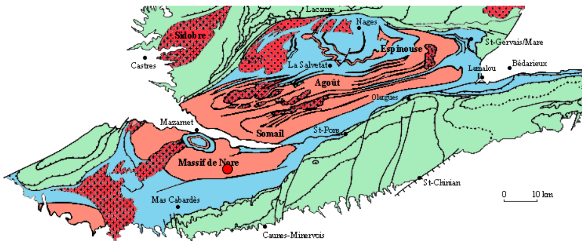
Figure 4 : Schéma structurel général de la Zone axiale de la Montagne Noire (d'après Demange1997).
